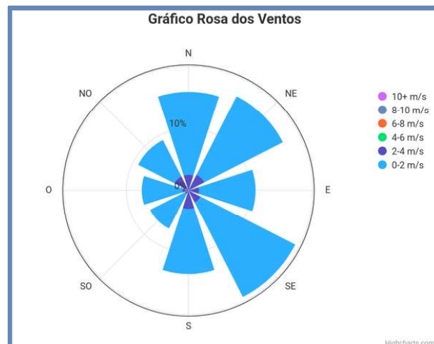
Gráfico 6 - Gráfico Rosa dos Ventos
