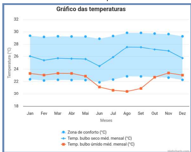
Gráfico 1 - Gráfico de Temperatura
