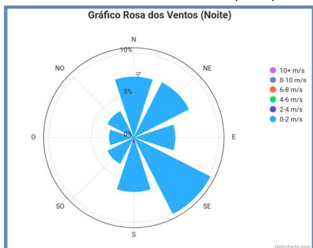
Gráfico 7 - Gráfico Rosa dos Ventos (Noite)
