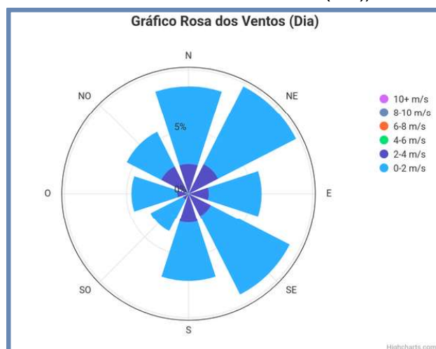
Gráfico 8 - Gráfico Rosa dos Ventos (Dia)
